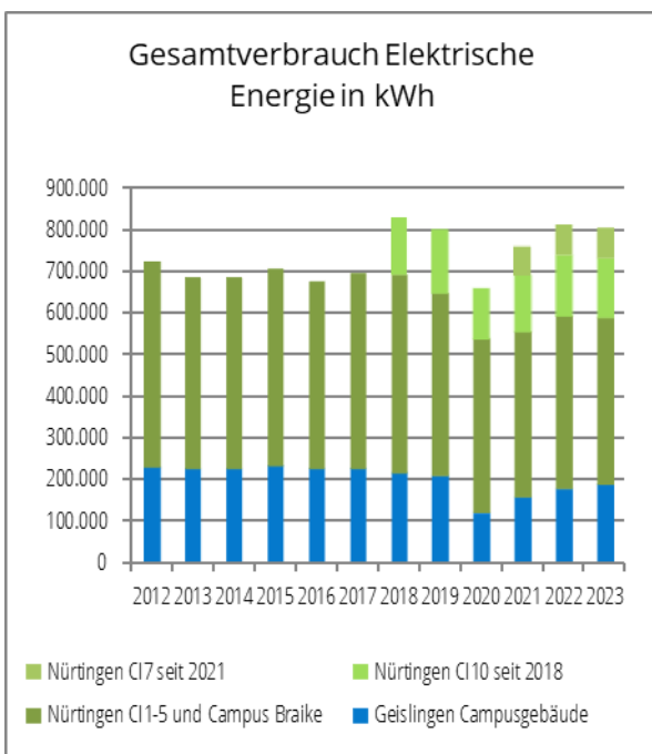
Abb. 18: Stromverbrauch der Campusgebäude
